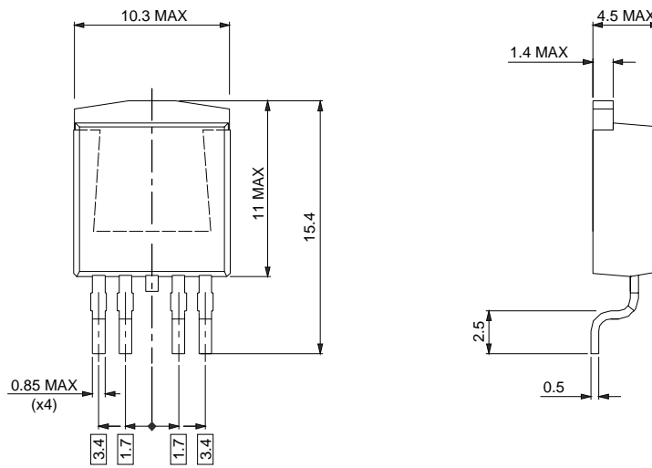
Fig.38. SOT426
