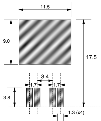
Fig.39. SOT426
