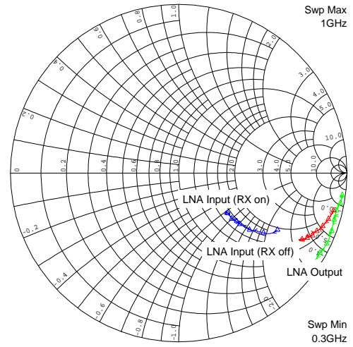
LNA Impedance
