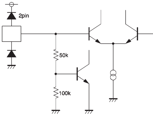
Op-amp input
