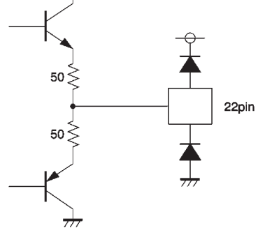
Op-amp output
