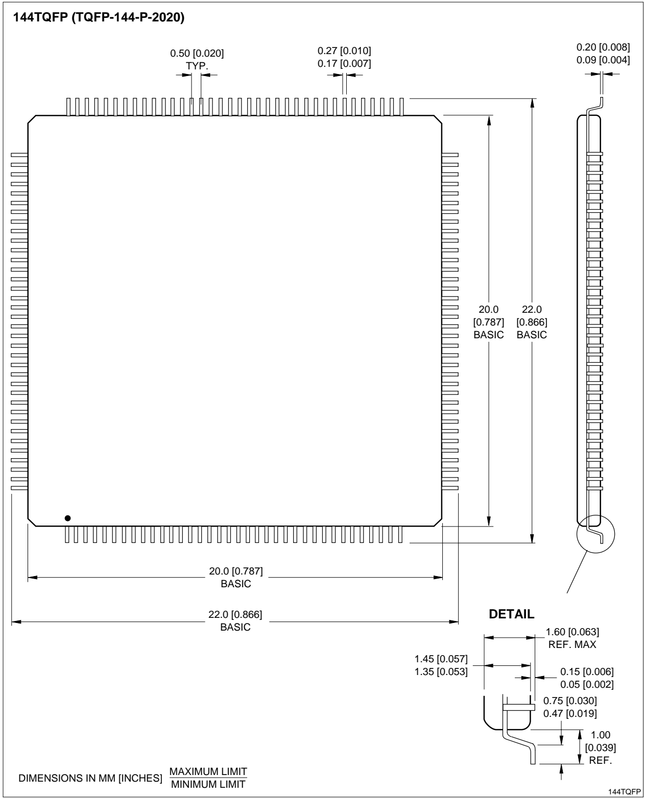
144-pin TQFP
