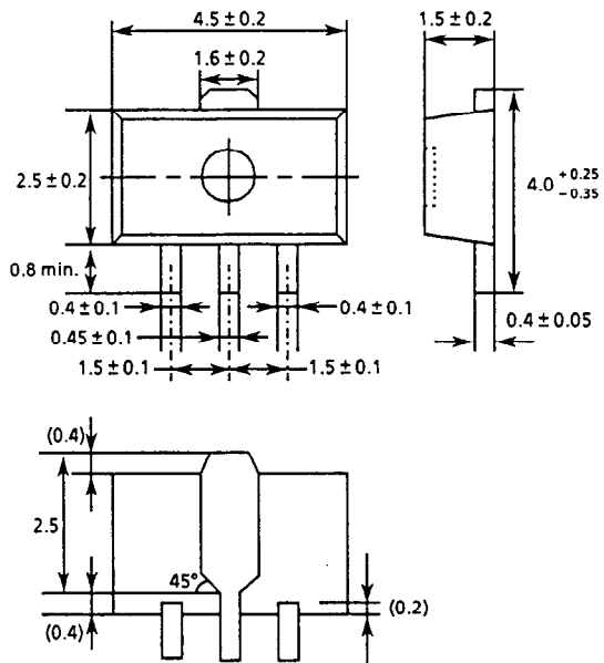
(2) SOT-89-3
