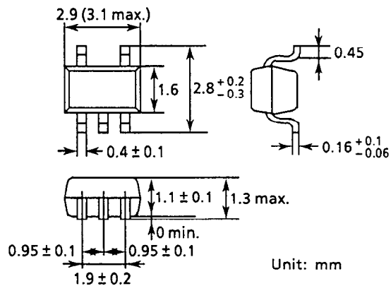
(3) SOT-23-5
