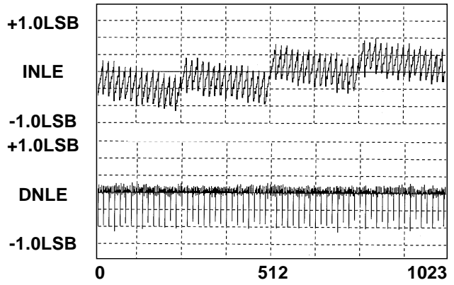
Vcc = 3.30V
