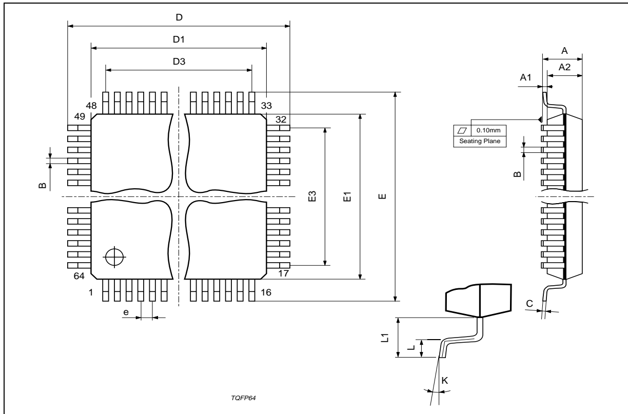
TQFP64
