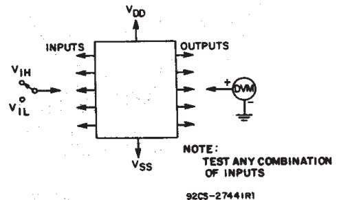
Fig. 14 - Input voltage.
