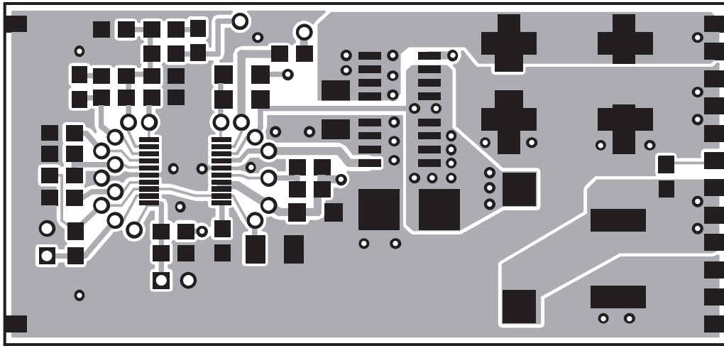
Top Layer
