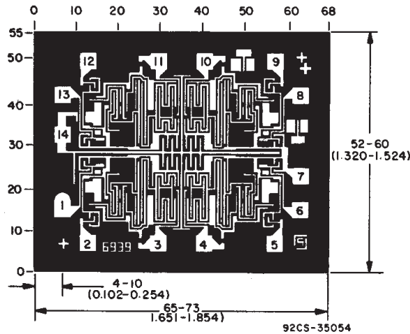
CD4001B
