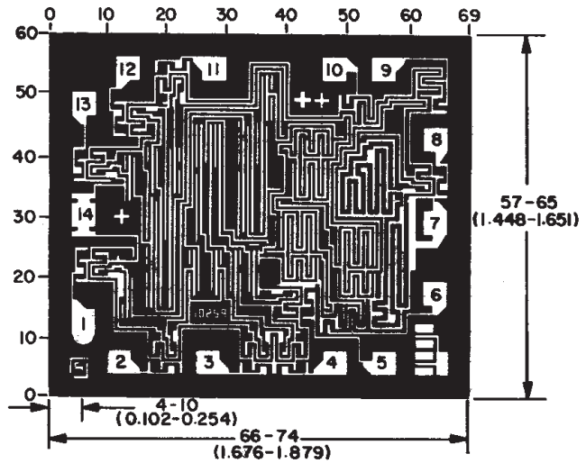
CD4025B
