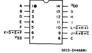
CD4025B
