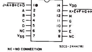
CD4002B
