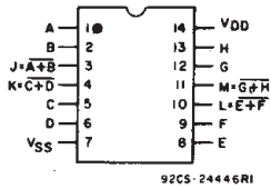
CD4001B
