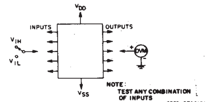
Fig. 18 - Input voltage test circuit.
