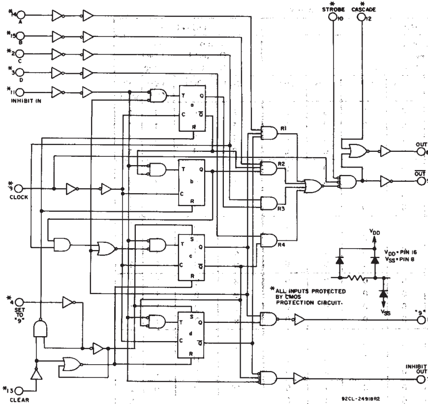
Fig. 13 - Logic diagram.
