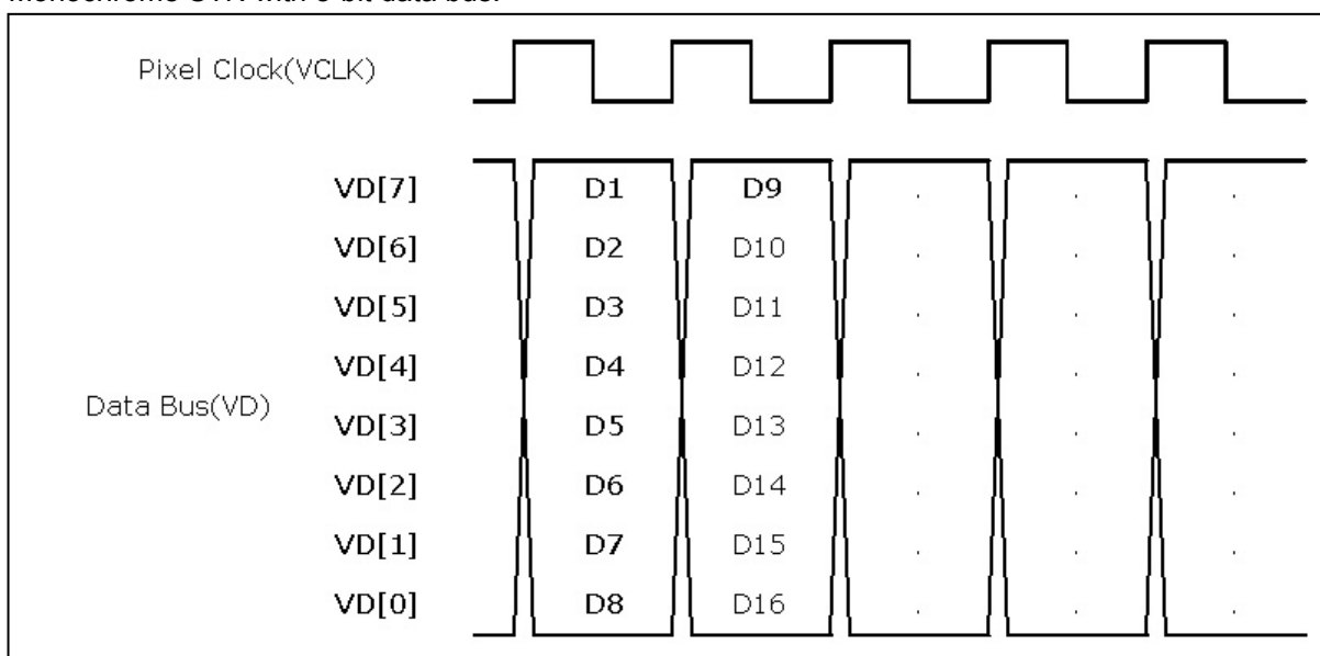
Fig. 6.10.3.6 Monochrome STN output format - 2
