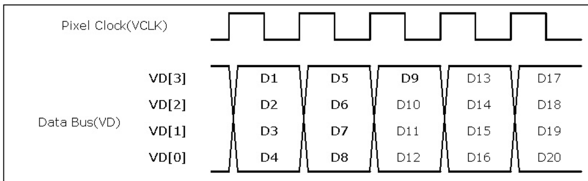
Fig. 6.10.3.5 Monochrome STN output format - 1
